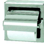
VDH BSB 096 F Tekli tuvalet kağıt dispenseri, siva üstü, parlak çelik gövde, tek rulo kapasiteli, duvara monteli. Ebat:160x160x55mmh
